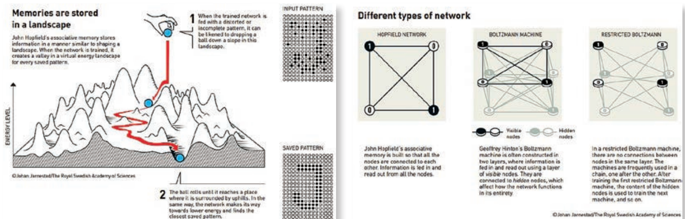
Slika 1: Hopfieldove mreže pohranjuje obrasce kao stabilna stanja minimalne energije. Preuzeto: Press release: The Nobel Prize in Physics 2024 - NobelPrize.org
